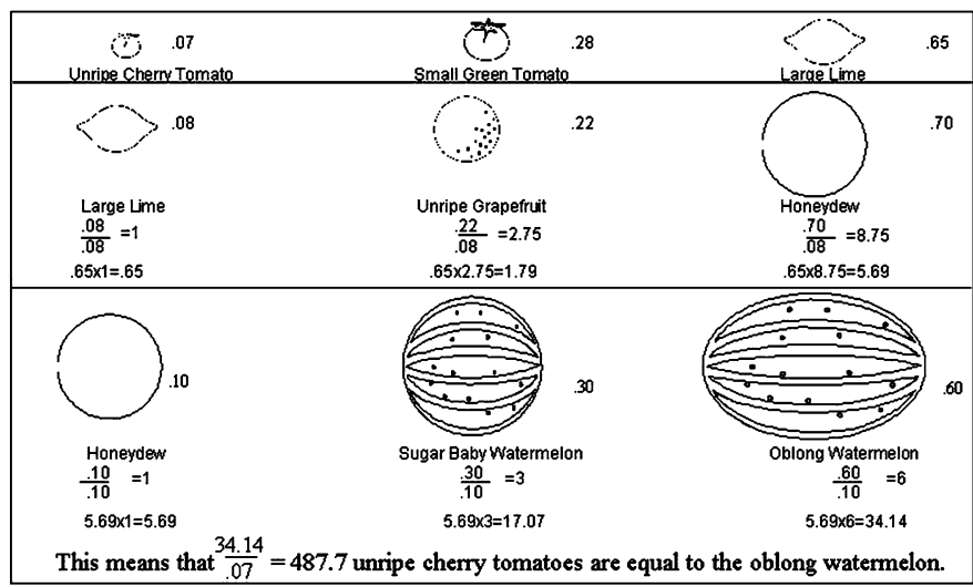
Fig. 2.1 Clustering
